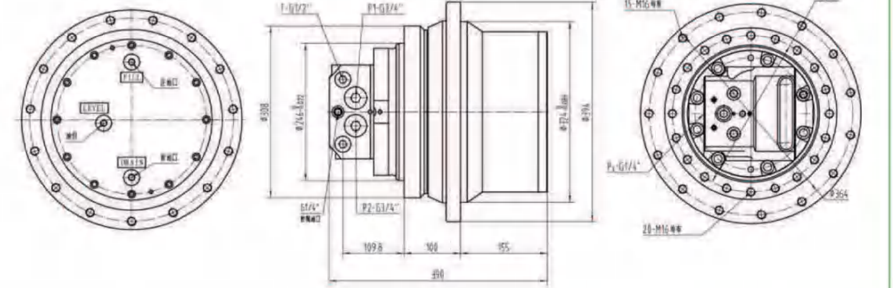
TM18B总装外形图
