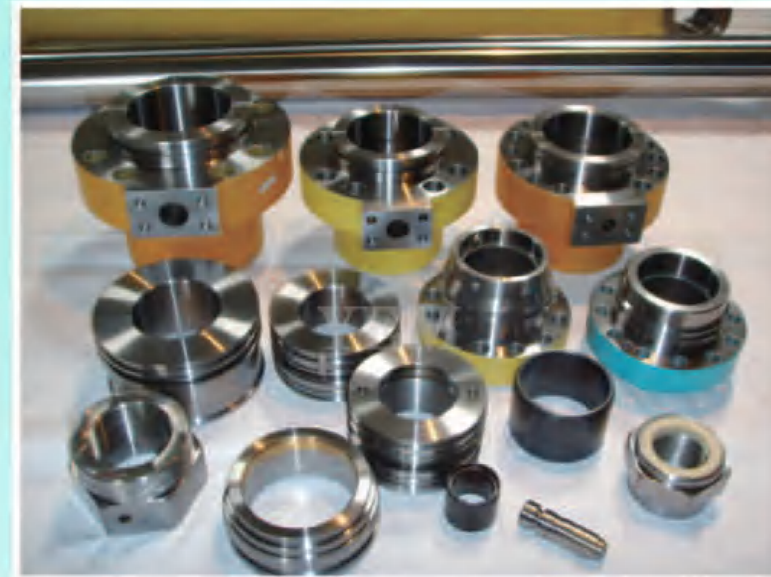
缸盖、活塞、螺母、前后缓冲
