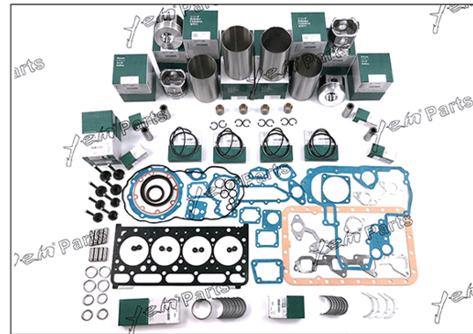
YEM-H8649 D7E组件
