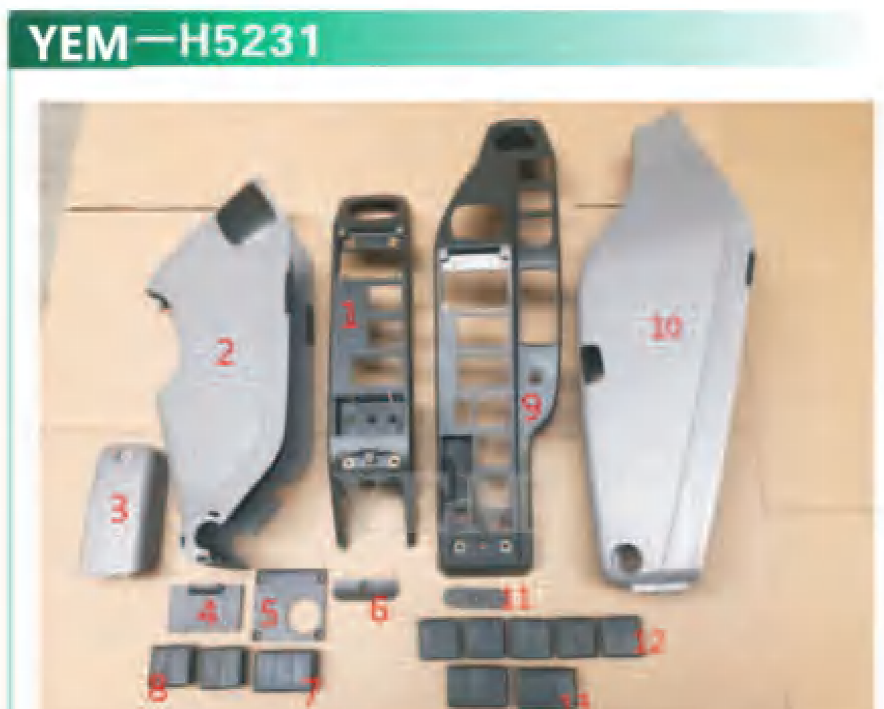
沃尔沃480D扶手箱
