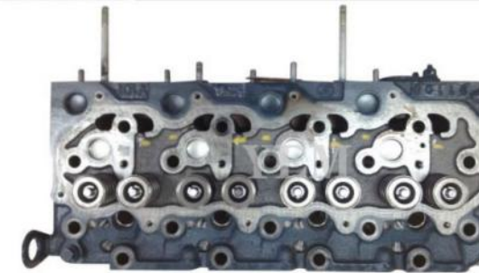
PC56-7 V2403 (1)
