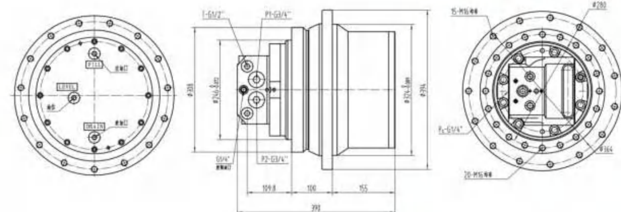
TM18B总装外形图
