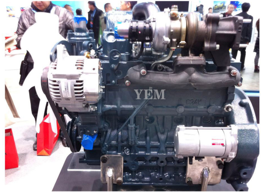
KUBOTA V2403
